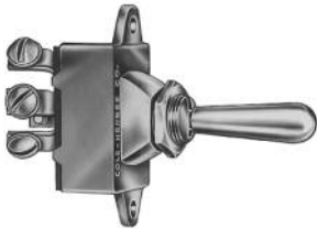
M-3034 SHOWN
